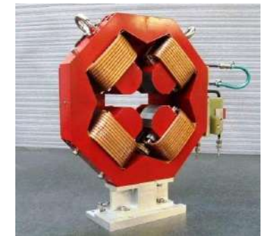
QUADRUPOLO
